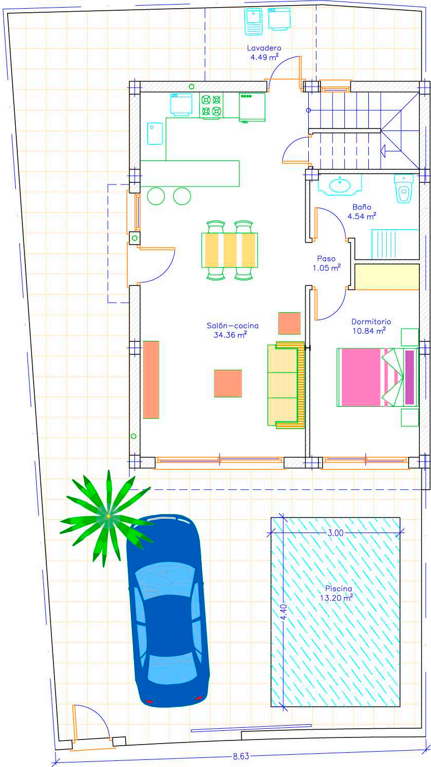
PLANTA BAJA
