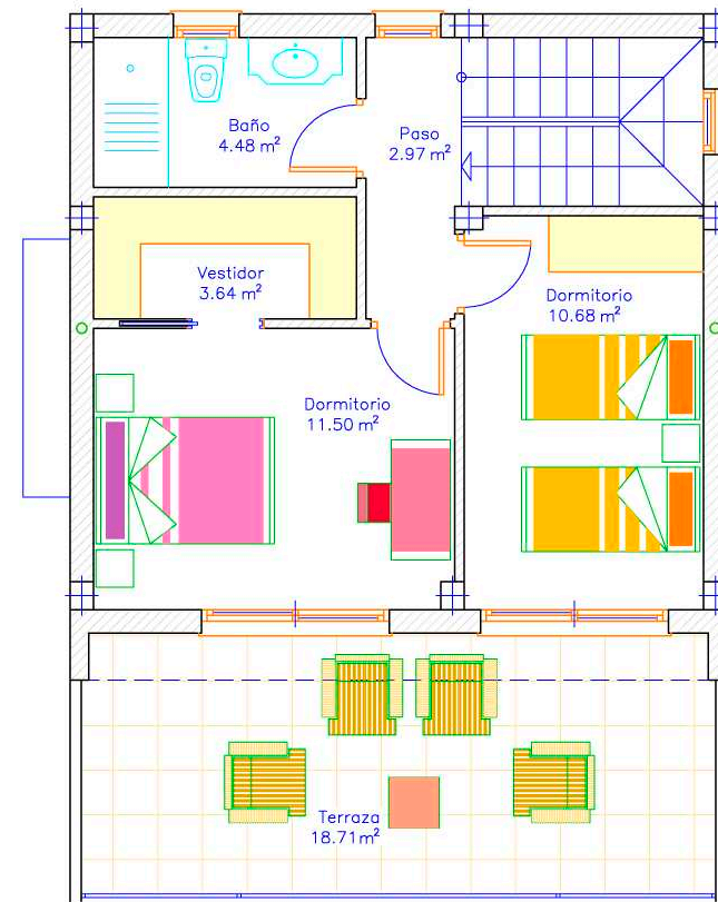
PLANTA ALTA
